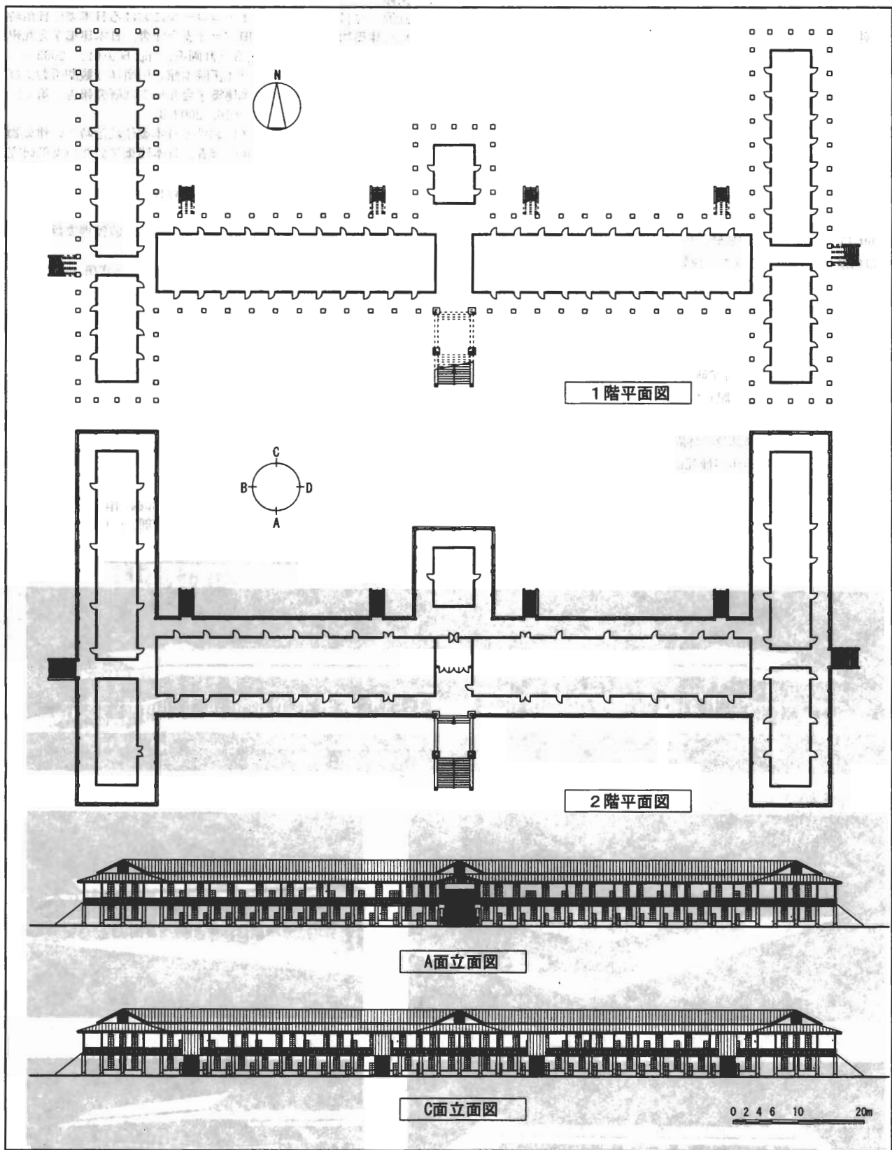
図1 南洋庁本庁庁舎復元図
