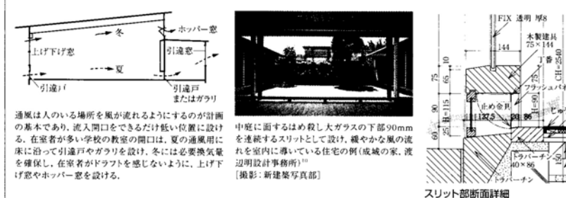
通風輪道の確保 04 [6] ⇨ 環境編 ⑥: 通風計画・設計諸例
