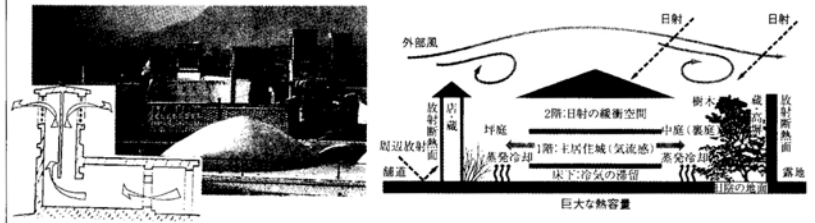
日射が塔が熱せられ、室内の暖かい空気が上昇し、涼しい空気が引き込まれる。高温乾燥地域で換気塔を備え、家の中に風道を作っている例。
