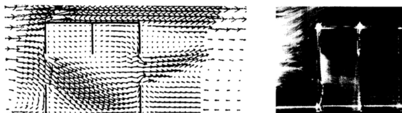
風の流れを確かめる 05 [4] ⇨ 環境編 ⑥: 室内気流数値計算プログラム
