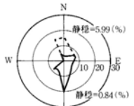
時間帯別風配
