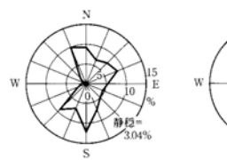
東京における蒸暑季(日平均気温 \geq 20 ℃、5月下旬~10月初旬)は、大洋から大陸に吹き込む季節風と海陸風が頻りに発達する。風向を時間帯別すると、卓越風向がより明確になる。季節風と海風の風向が一致する時間帯の風速は、陸寄りの風が吹く時間帯に比較して1.5倍程度大きい。
