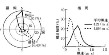
蒸暑季の大阪(5月中旬~10月初旬)と福岡(5月中旬~10月中旬)における時間帯別風配と風速頻度分布 大阪:実線は13:00~18:00、破線は3:00~8:00のデータ。福岡:実線は12:00~18:00、破線は24:00~6:00のデータ
