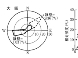
蒸暑季の大阪(5月中旬~10月初旬)と福岡(5月中旬~10月中旬)における時間帯別風配と風速頻度分布 大阪:実線は13:00~18:00、破線は3:00~8:00のデータ。福岡:実線は12:00~18:00、破線は24:00~6:00のデータ
