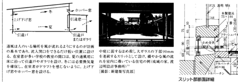
通風は人のいる場所を風が流れるようにするのが計画の基本であり、流入開口をできるだけ低い位置に設ける。在室者が多い学校の教室の開口は、夏の通風用に床に沿って引違戸やガラリを設け、冬には必要換気量を確保し、在室者がドラフトを感じないように、上げ下げ窓やホッパー窓を設ける。 中庭に面するはめ殺し大ガラスの下部90mmを連続するスリットとして設け、緩やかな風の流れを室内に導いている住宅の例(成城の家、渡辺明設計事務所) [撮影: 新建築写真部] スリット断面詳細
