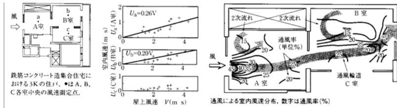
鉄筋コンクリート造集合住宅における3Kの住戸。●はA, B, C各室中央の風速測定点。 屋上風速 V (m/s) 室内風速 U a (A室) U a (B室) U a (C室) 屋上風速 V と室内風速 U の関係 通風による室内風速分布。数字は通風率(%)
