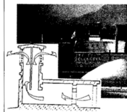
日射が塔が熱せられ、室内の暖かい空気が上昇し、涼しい空気が引き込まれる。高温乾燥地域で換気塔を備え、家の中に風道を作っている例。
