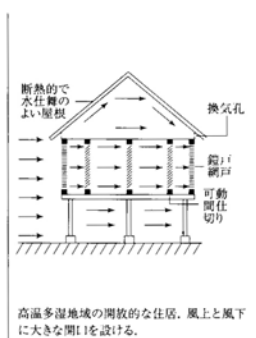
高温多湿地域の開放的な住居。風上と風下に大きな開口を設ける。
