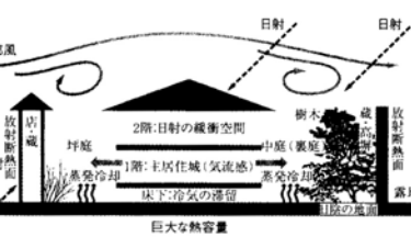
植栽や水面を有して低温面を形成する二つの中庭の空間ボリュームの違いによって生じる圧力差を利用し、室内に風を発生させ、深い軒庇、葺や高層によって日射を遮蔽している京都の町家。
