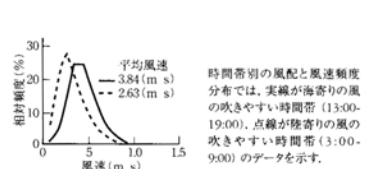
時間帯別の風配と風速頻度分布では、実線が海寄りの風の吹きやすい時間帯(13:00-19:00)、点線が陸寄りの風の吹きやすい時間帯(3:00-9:00)のデータを示す。
