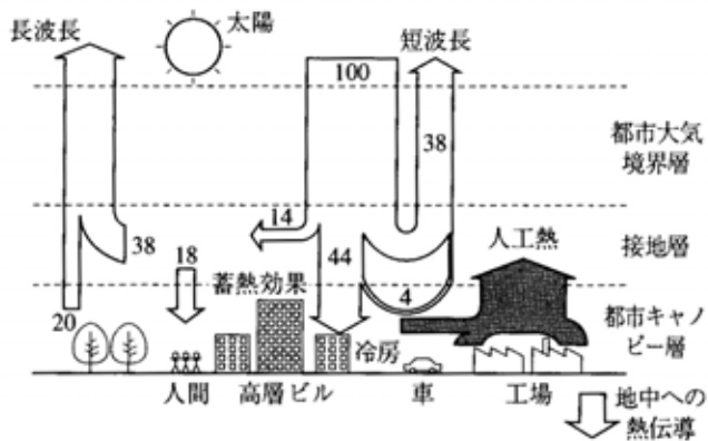
図 都市大気熱の熱バランス (出典：参考文献 [3], p. 64)
